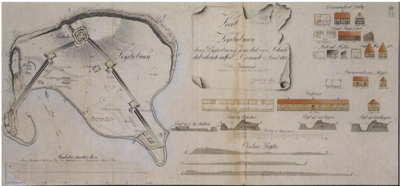
Projekt til forsvarsanlæg på Kyholm, udført af infanterikaptajn Nicolaj Tidemand o. 1801
