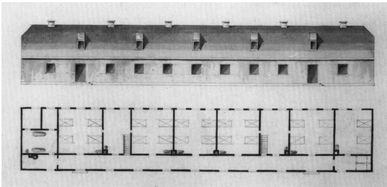
Plan og opstalt af sygehuset på Kyholm i karantænetiden 1831 - 59. Kapellet var sandsynligvis indrettet i den stue, der på tegningen rummer to senge. Tegning af Jørgen Hansen Koch 1831.
